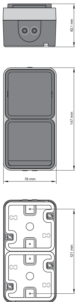
Afbeelding 13: Combinatie wisselchakelaar/wandcontactdoos met klapdeksel
